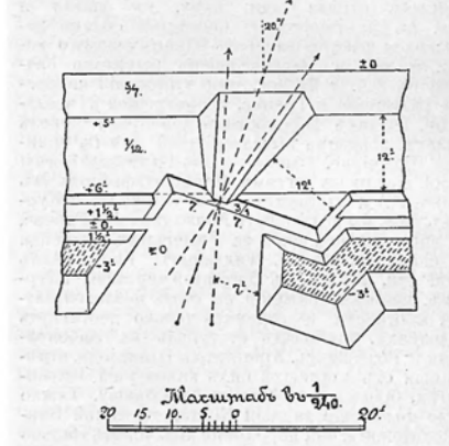
Косая амбразура.
